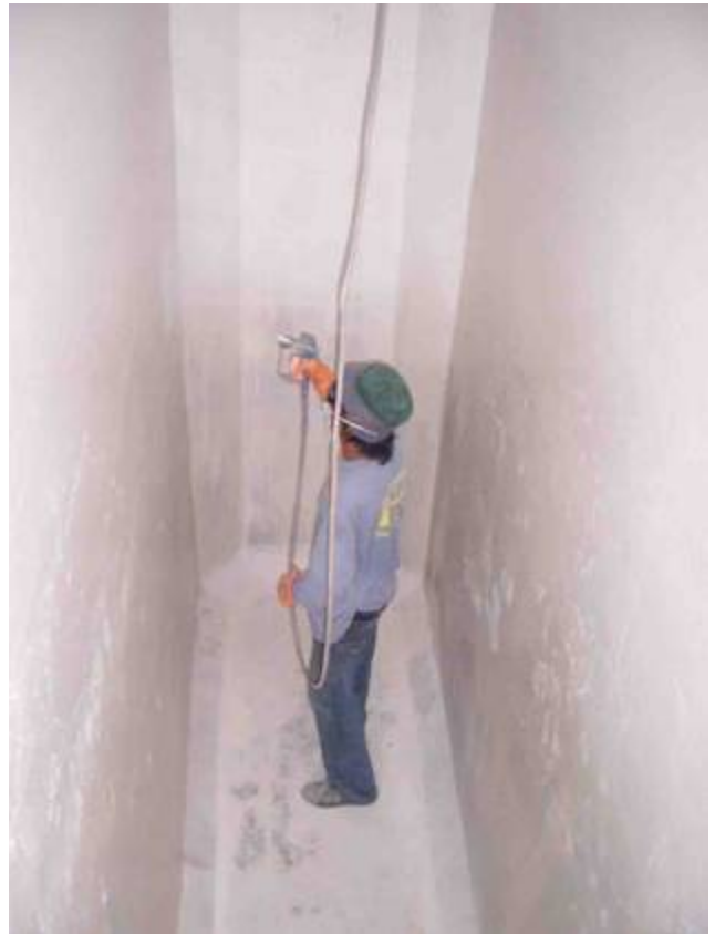
พ่นสีอิพ็อกซี Hydrocote เทียวที่ 2 และ 3
